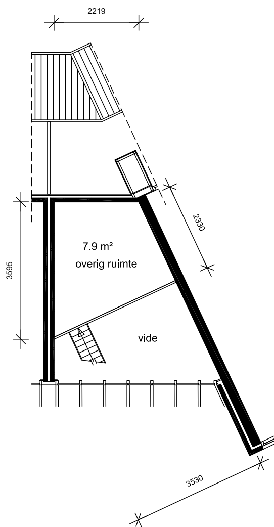
PLATTEGROND (zolder)
