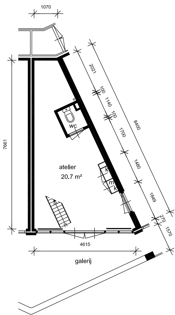
PLATTEGROND (3e. verdieping)
