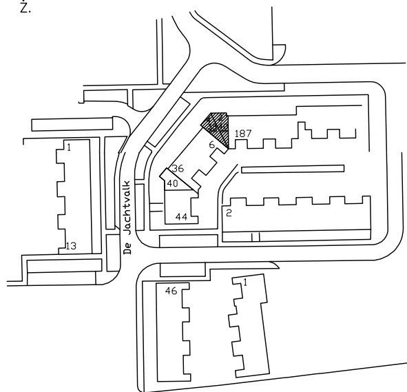
SITUATIE (1:2000)
